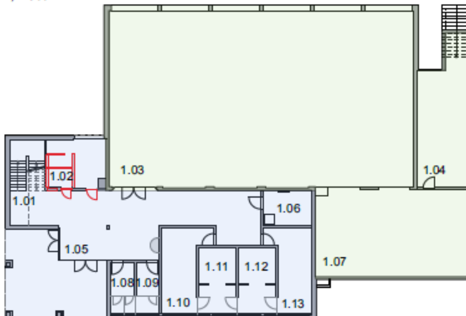
Grundriss EG M, 1:300
